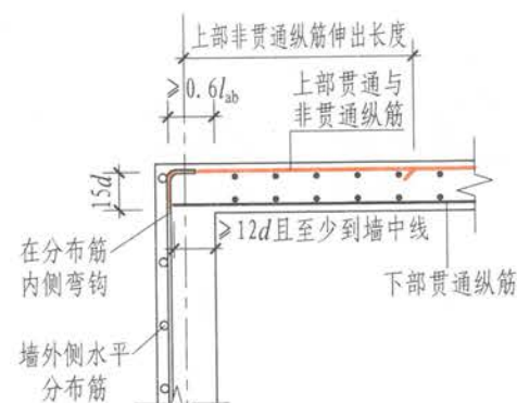
(2) 板端上部纵筋按充分利用钢筋的抗拉强度时
