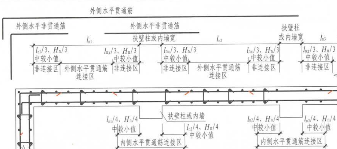
地下室外墙水平钢筋构造
