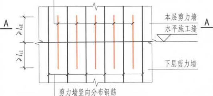
施工缝处抗剪用钢筋连接构造
