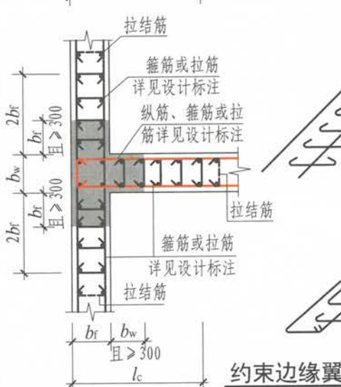
约束边缘翼墙 (一)
