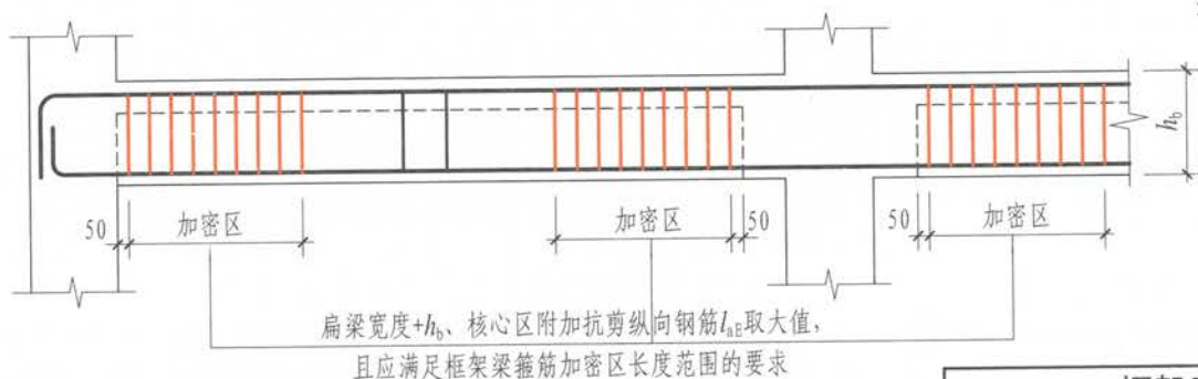
框架扁梁箍筋构造
