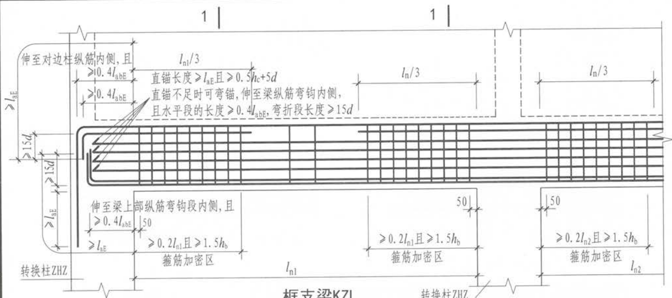
框支梁KZL (也可用于托柱转换梁TZL)
