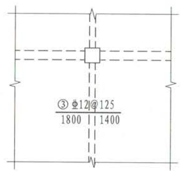
图5.3.1-2 板支座上部非贯通纵筋非对称伸出
