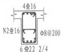
1-1 300 × 550
