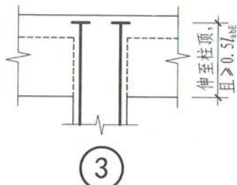
柱纵向钢筋端头加锚头(锚板)
