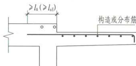
仅上部配筋
