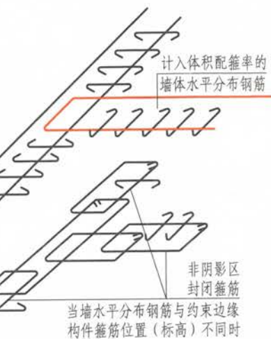
约束边缘翼墙 (一)
