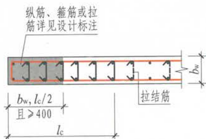
约束边缘暗柱 (一)
