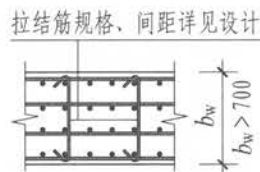
剪力墙四排配筋
