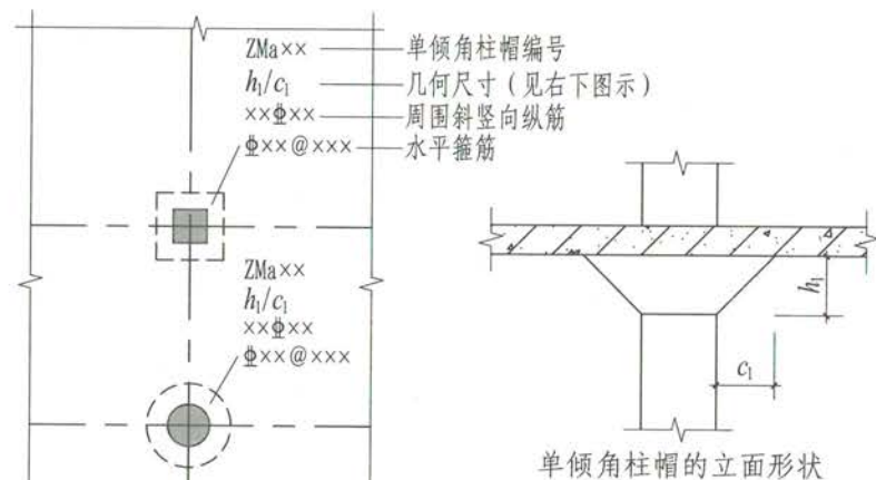
图7.2.3-1 单倾角柱帽ZMa引注图示
