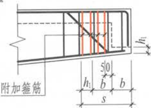
悬挑梁端附加箍筋范围
