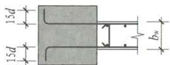
端柱端部墙 (一)
