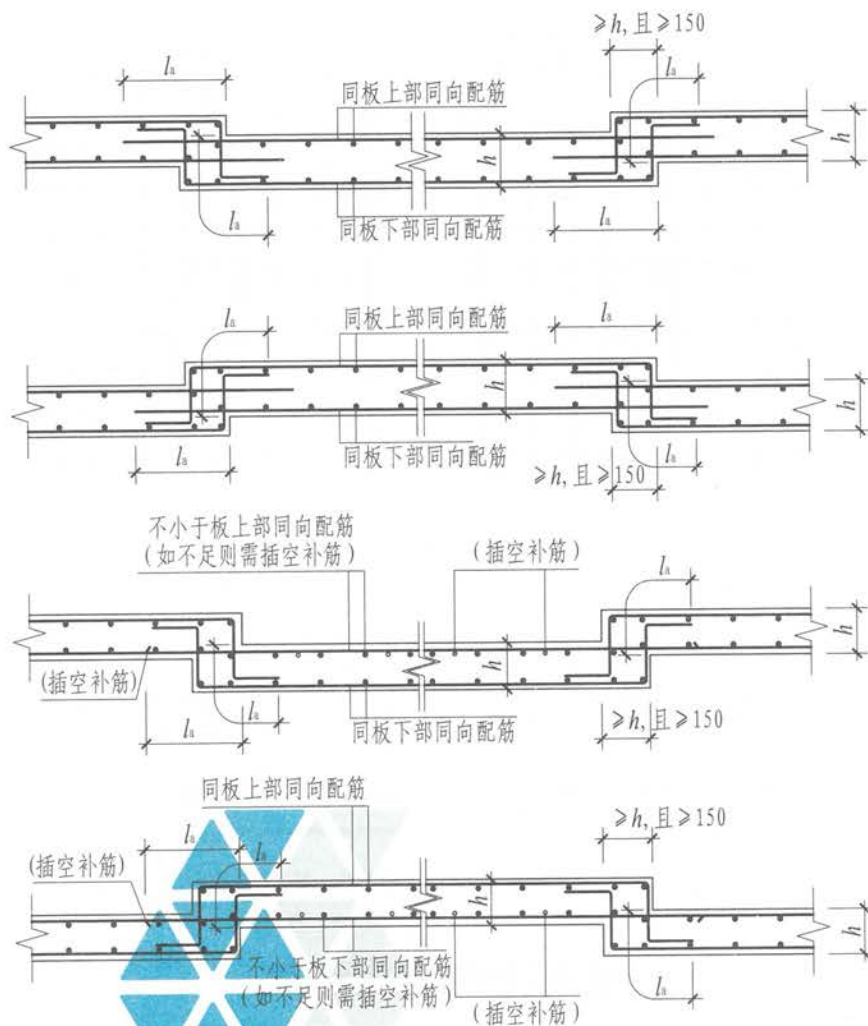
局部升降板SJB构造(二)
