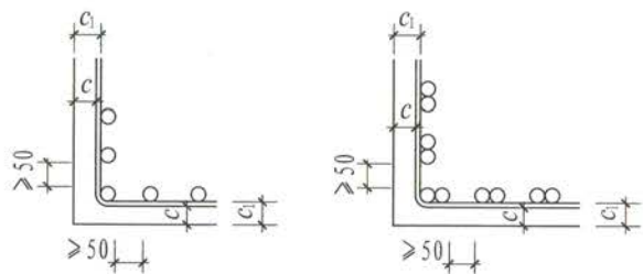
梁上部纵筋间距要求
