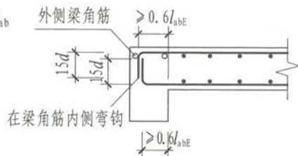
(b) 梁板式转换层的楼面板
