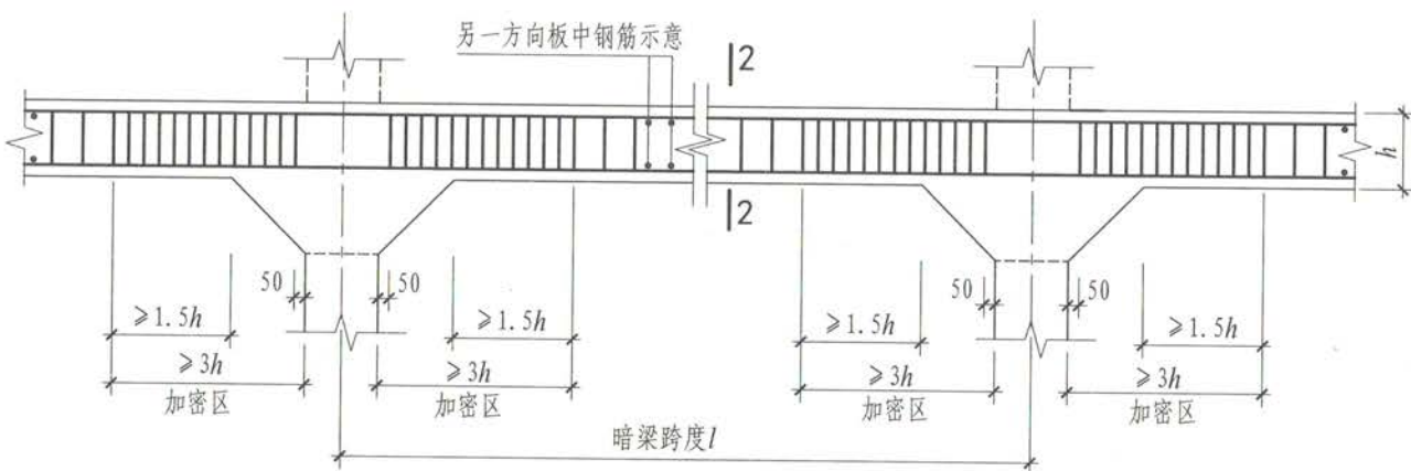
有柱帽柱上板带暗梁钢筋构造
