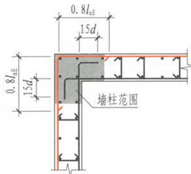
转角墙(三) (外侧水平分布钢筋在转角处搭接)
