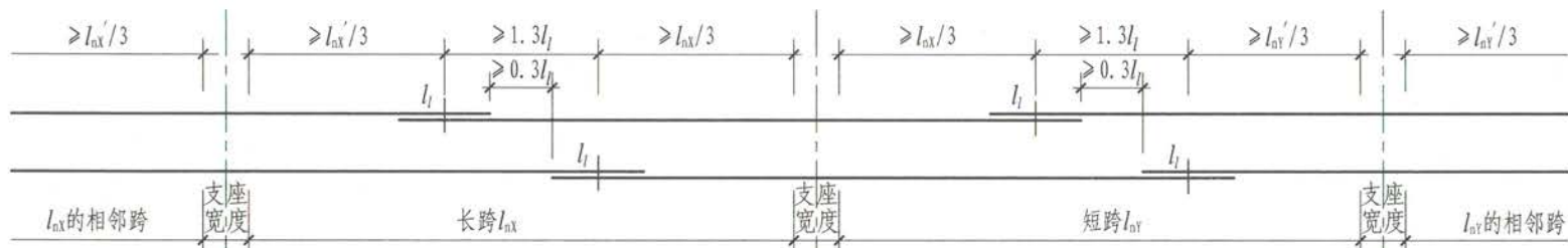
(A) 不等跨板上部贯通纵筋连接构造(一)
