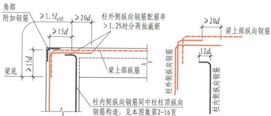
(b) 梁宽范围内钢筋
