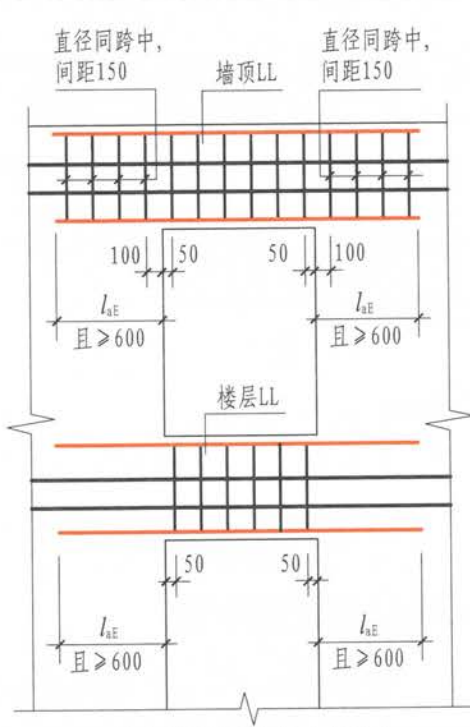
(b) 单洞口连梁 (单跨)
