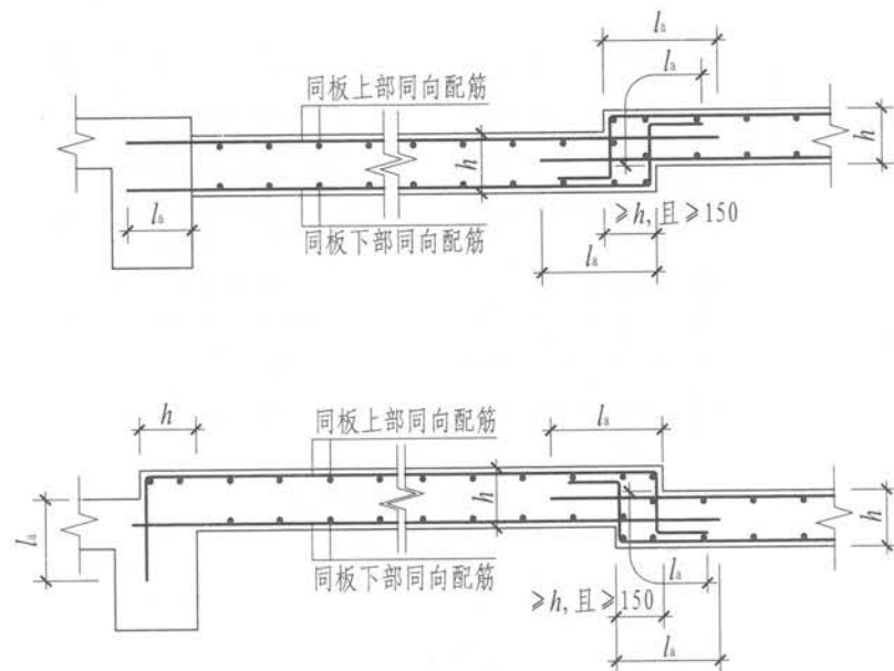
局部升降板SJB构造(二)
