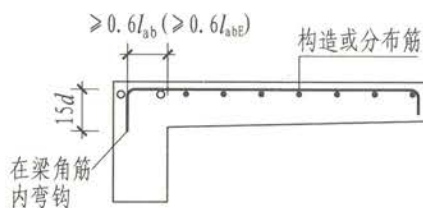
仅上部配筋
