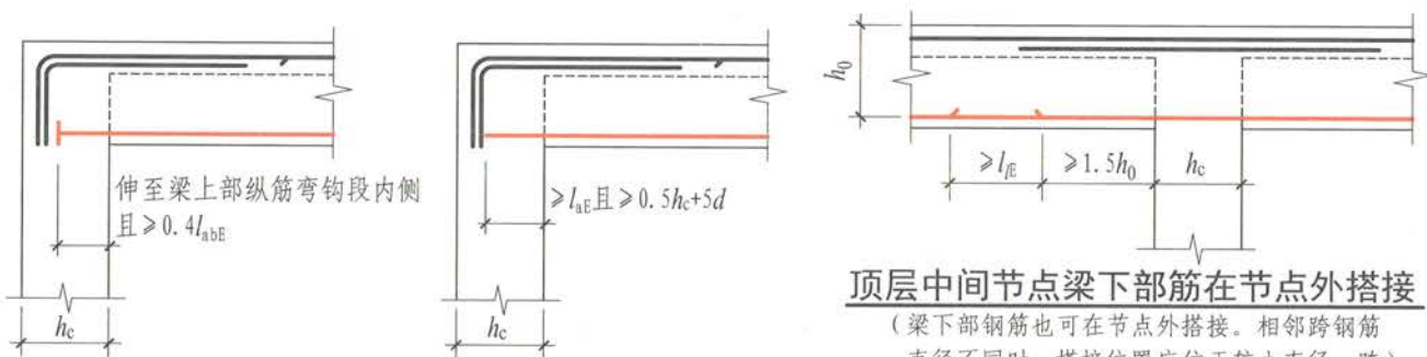
屋面框架梁WKL纵向钢筋构造
