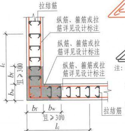
约束边缘转角墙
