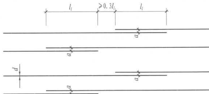
纵向钢筋非接触搭接构造
