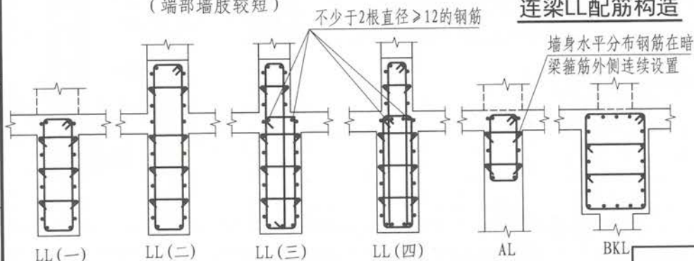
连梁、暗梁和边框梁侧面纵筋和拉筋构造
