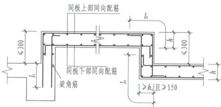
局部升降板SJB构造(一)
