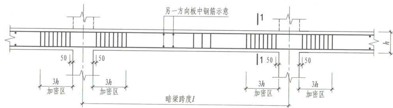
无柱帽柱上板带暗梁钢筋构造
