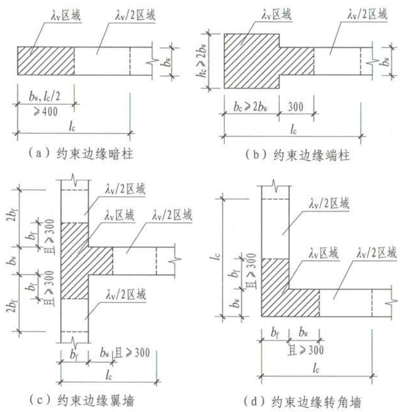
图3.2.2-2 约束边缘构件
