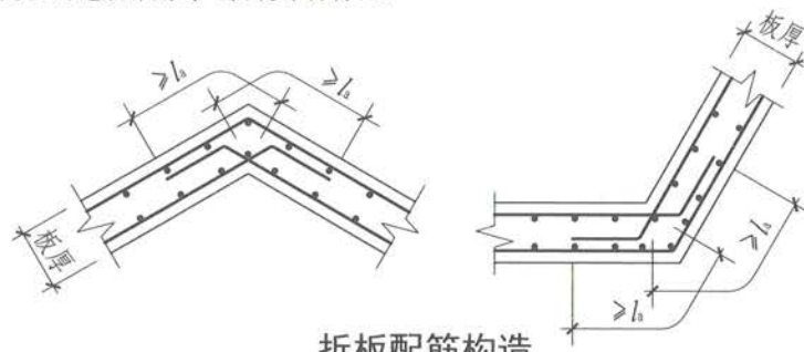
折板配筋构造
