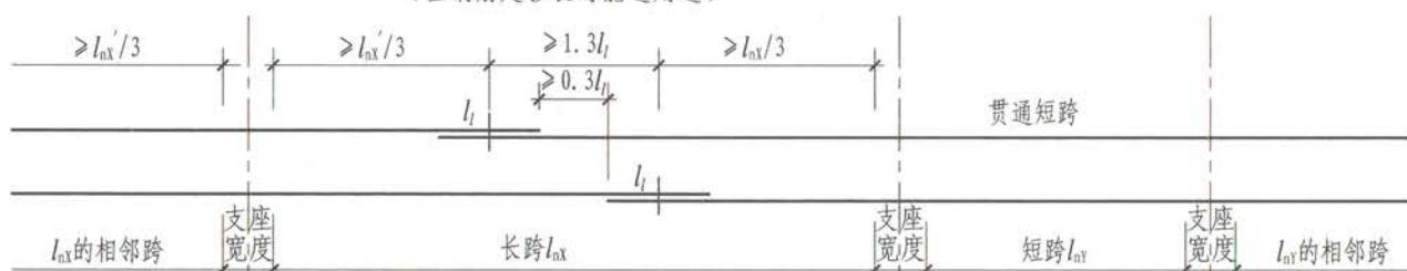
(A) 不等跨板上部贯通纵筋连接构造(三)
