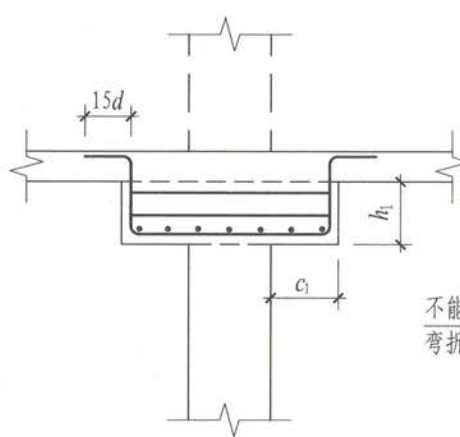
托板柱帽ZMb构造
