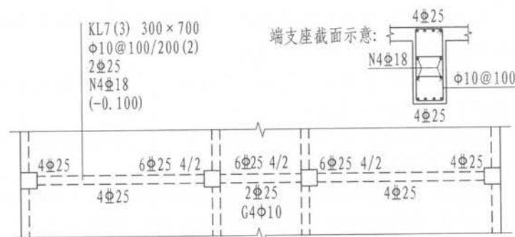
图4.2.4-1 大小跨梁的注写示例
