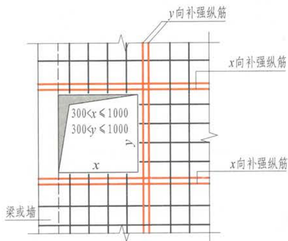
(b) 梁边或墙边开洞
