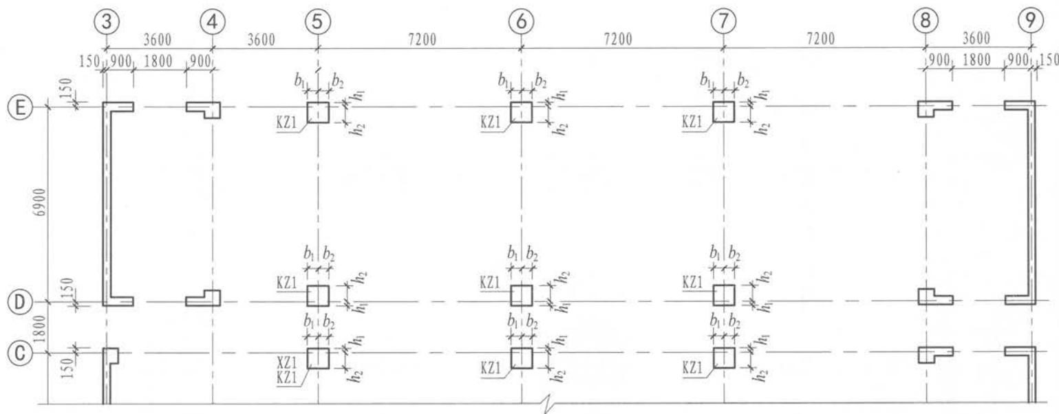
柱表
