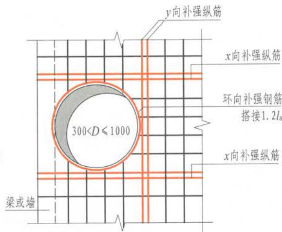
(b) 梁边或墙边开洞
