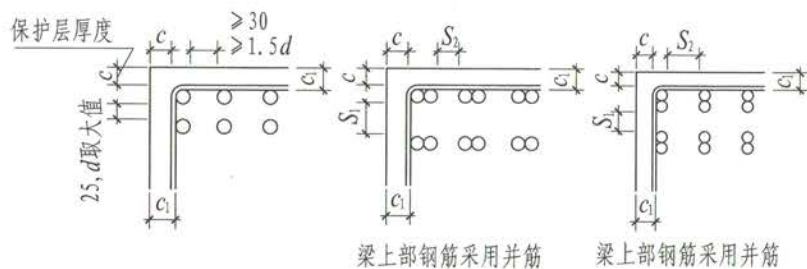
梁上部纵筋间距要求
