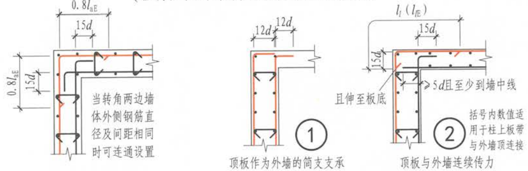
地下室外墙转角配筋构造
