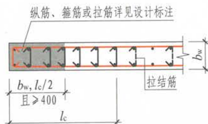
约束边缘暗柱 (二)
