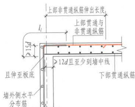
(1) 搭接连接
