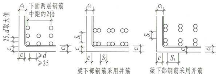
梁下部纵筋间距要求
