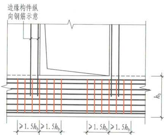
补强暗梁 设计指定
