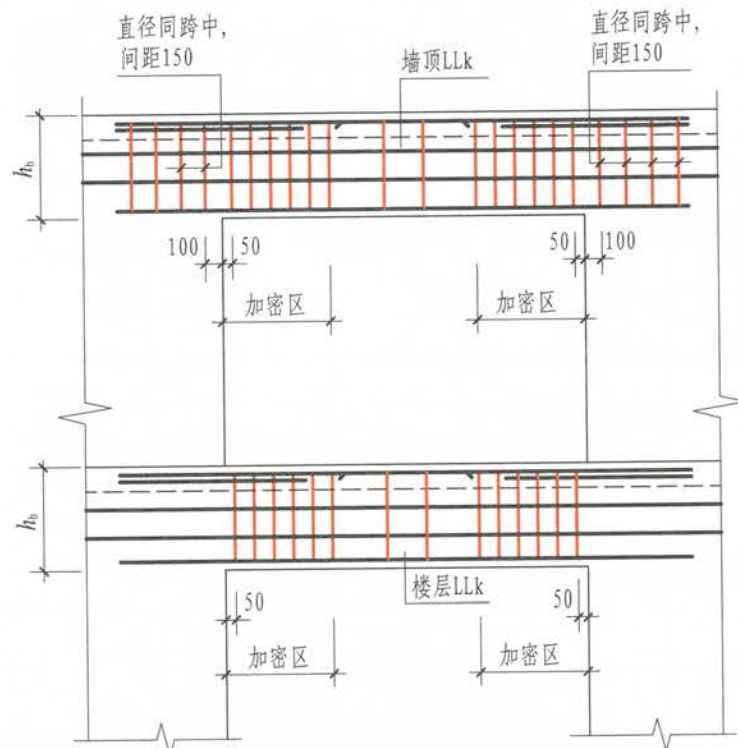
连梁LLk箍筋加密区范围
