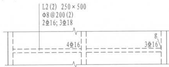
图4.2.4-5 梁一端采用充分利用钢筋抗拉强度方式的注写示意图 注:“g”表示右端支座按照非框架梁Lg配筋构造。
