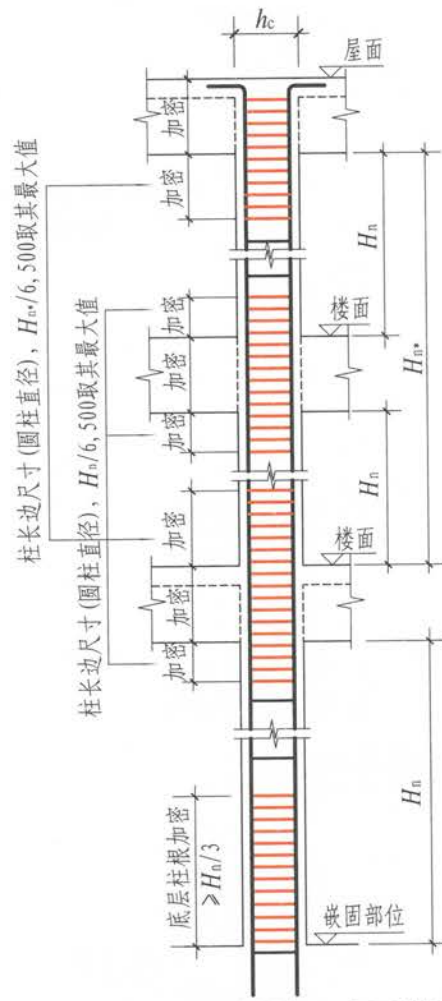
单向穿层KZ箍筋加密区范围 (单方向无梁且无板)
