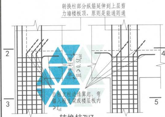
转换柱ZHZ (柱底纵筋的连接构造同抗震框架柱; 柱纵筋的连接宜采用机械连接接头)
