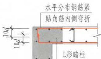
端部有L形暗柱时剪力墙水平分布钢筋端部做法
