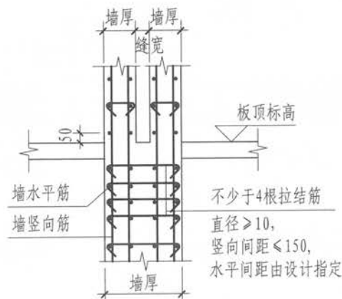
防震缝处墙局部构造
