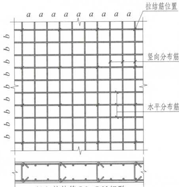
(b) 拉结筋@3a@3b矩形 (a ≤ 200, b ≤ 200)
