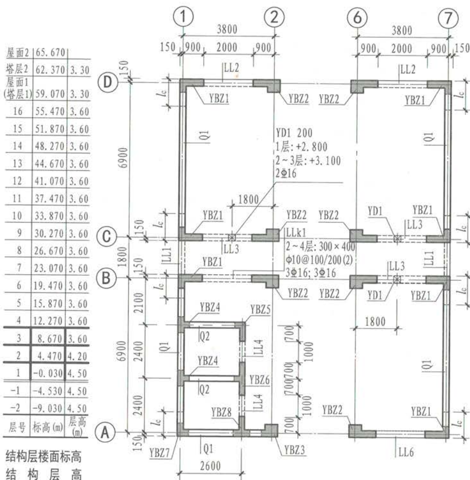
-0.030~12.270剪力墙平法施工图(局部)
