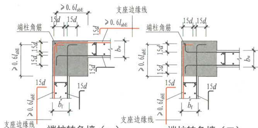
端柱转角墙 (一)
