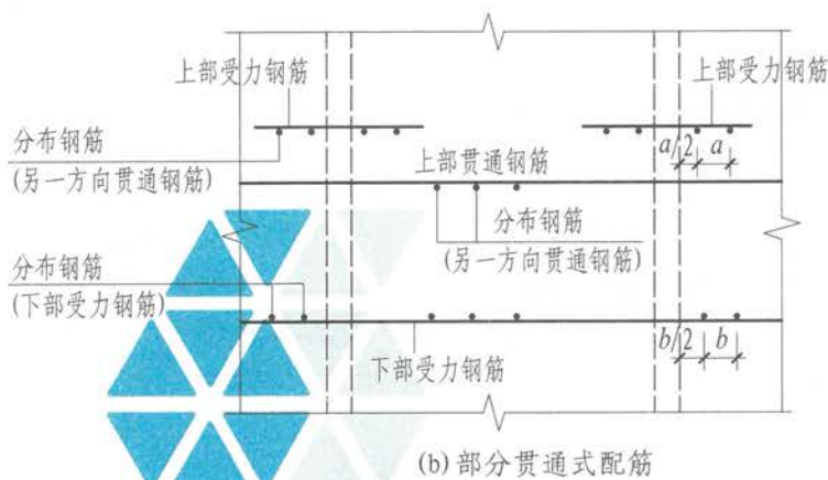
单（双）向板配筋示意
