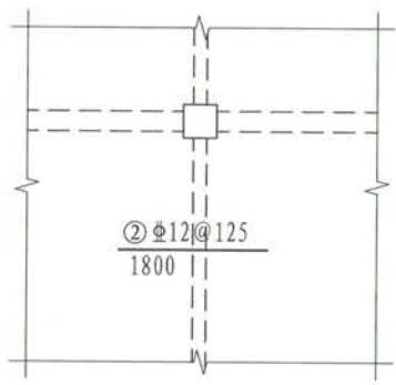
图5.3.1-1 板支座上部非贯通纵筋对称伸出
