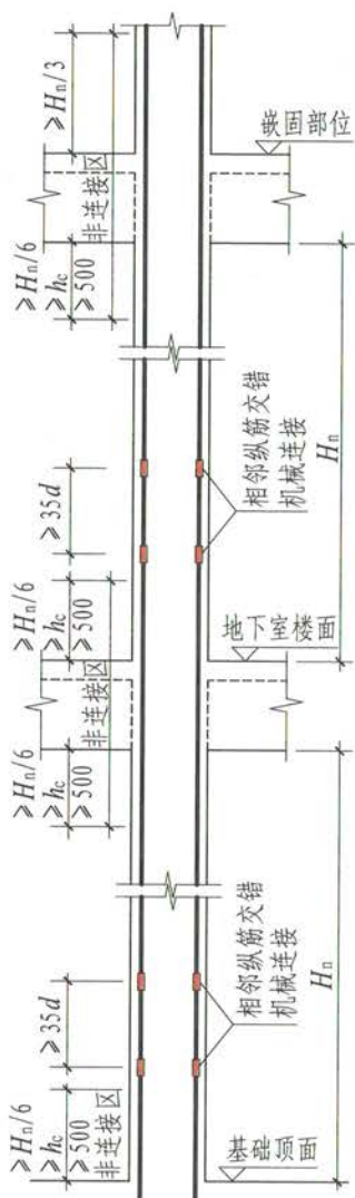
机械连接
