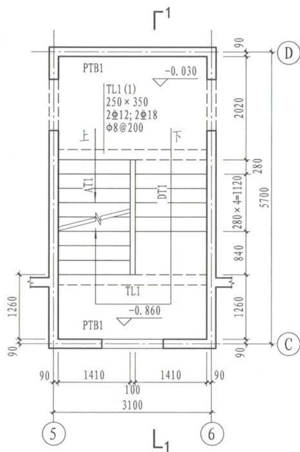
▽-0.860~▽-0.030楼梯平面图
