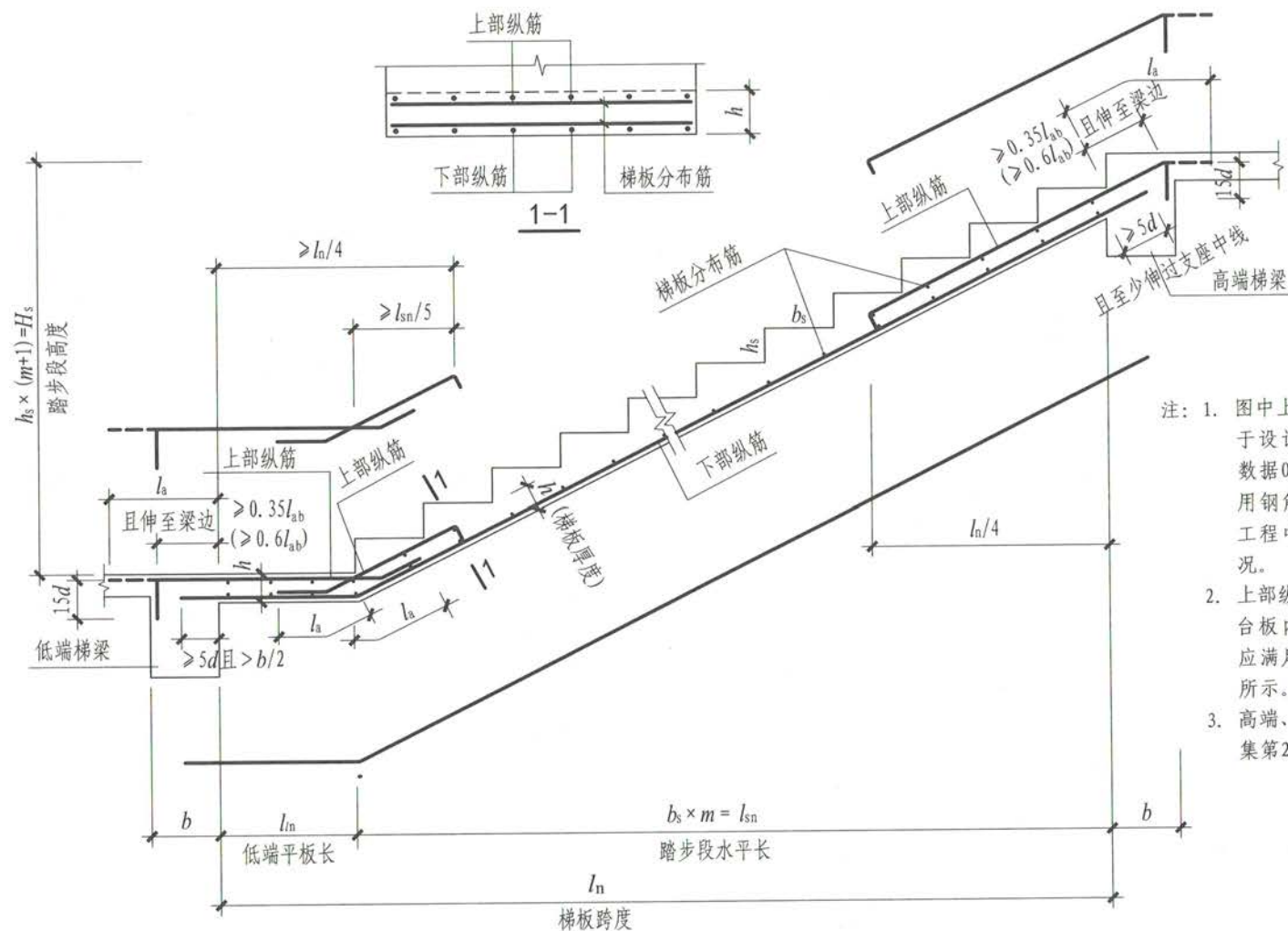
BT型楼梯板配筋构造
