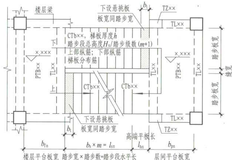
图2 \nabla x. \times \times \times \sim \nabla x. \times \times \times 楼梯平面图
