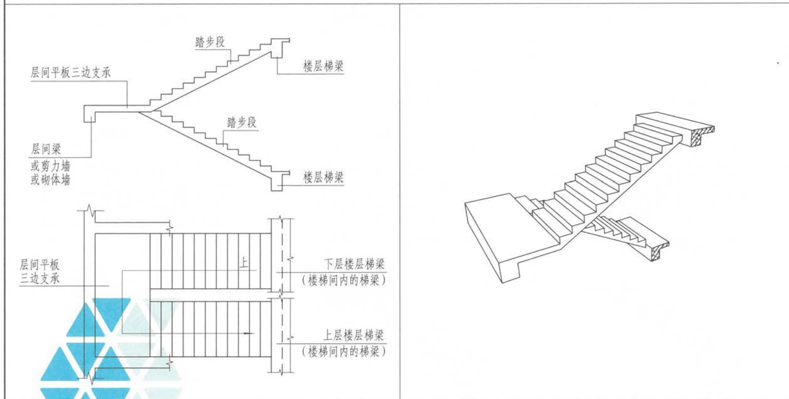
GT型楼梯截面形状与支座位置示意图
