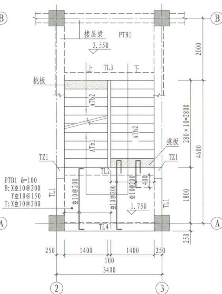
▽1.750~▽3.550楼梯平面图
