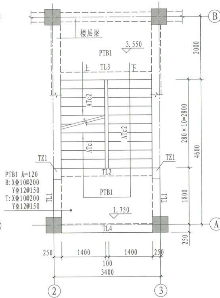
▽1.750~▽3.550楼梯平面图
