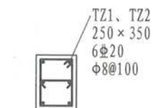
TZ1、TZ2
