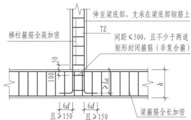
梁上立梯柱配筋构造 (一)
