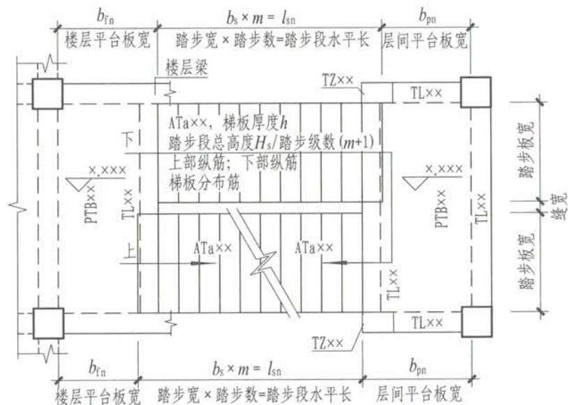
图1 \nabla x.xxx~ \nabla x.xxx楼梯平面图
