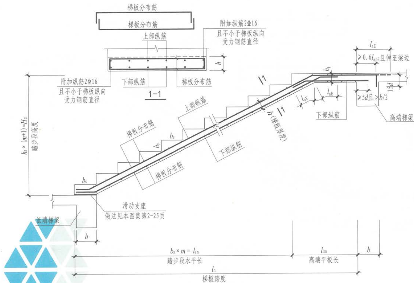
CTa型楼梯板配筋构造
