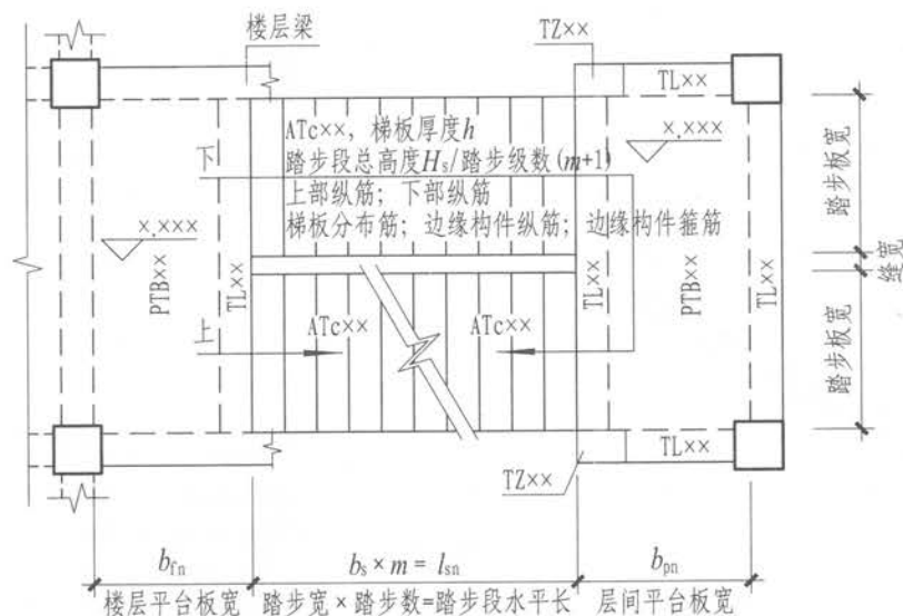
图1 \nabla x. xxx ~ \nabla x. xxx 楼梯平面图
