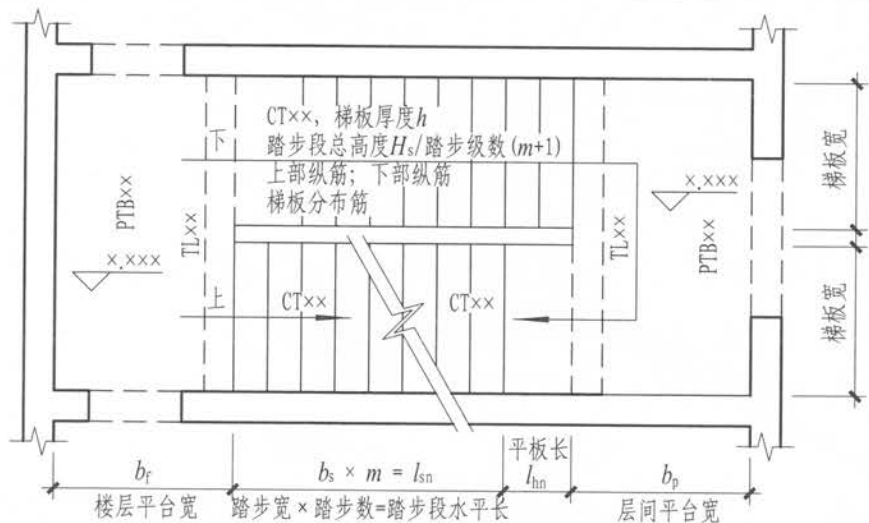
图1 \nabla x.xxx \sim \nabla x.xxx 楼梯平面图 (注写方式)
