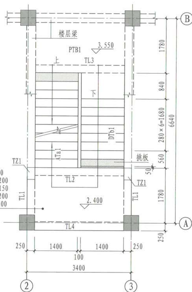
▽2.400~▽3.550楼梯平面图
