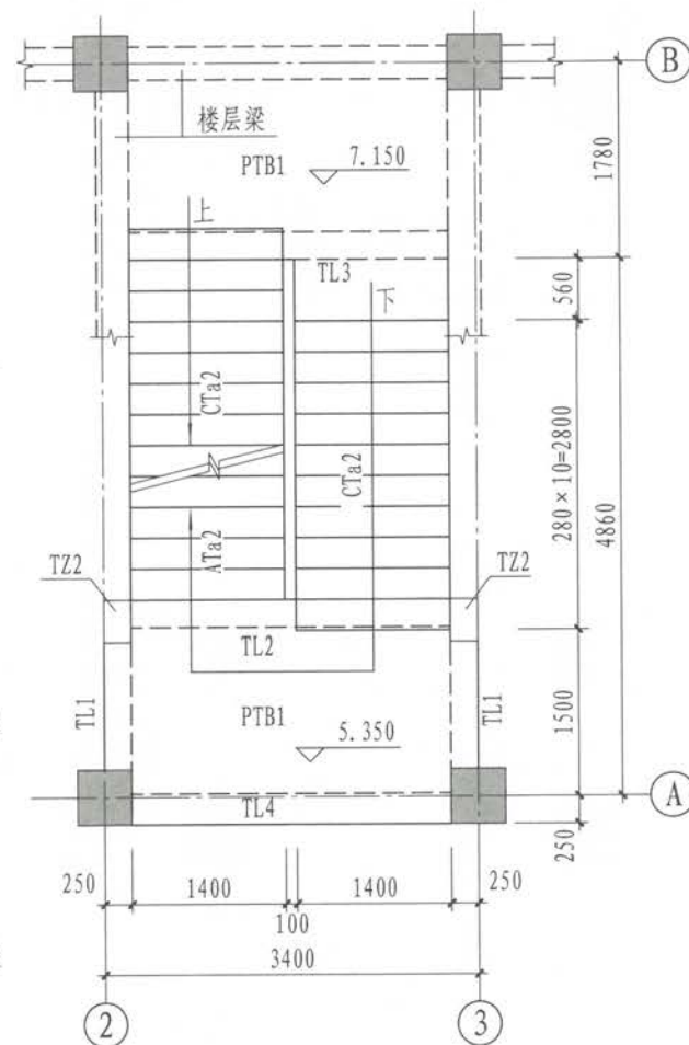
▽5.350~▽7.150楼梯平面图
