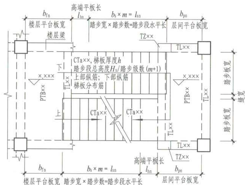
图1 \nabla x. \times \times \times \sim \nabla x. \times \times \times 楼梯平面图
