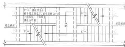
图4 剪刀楼梯
