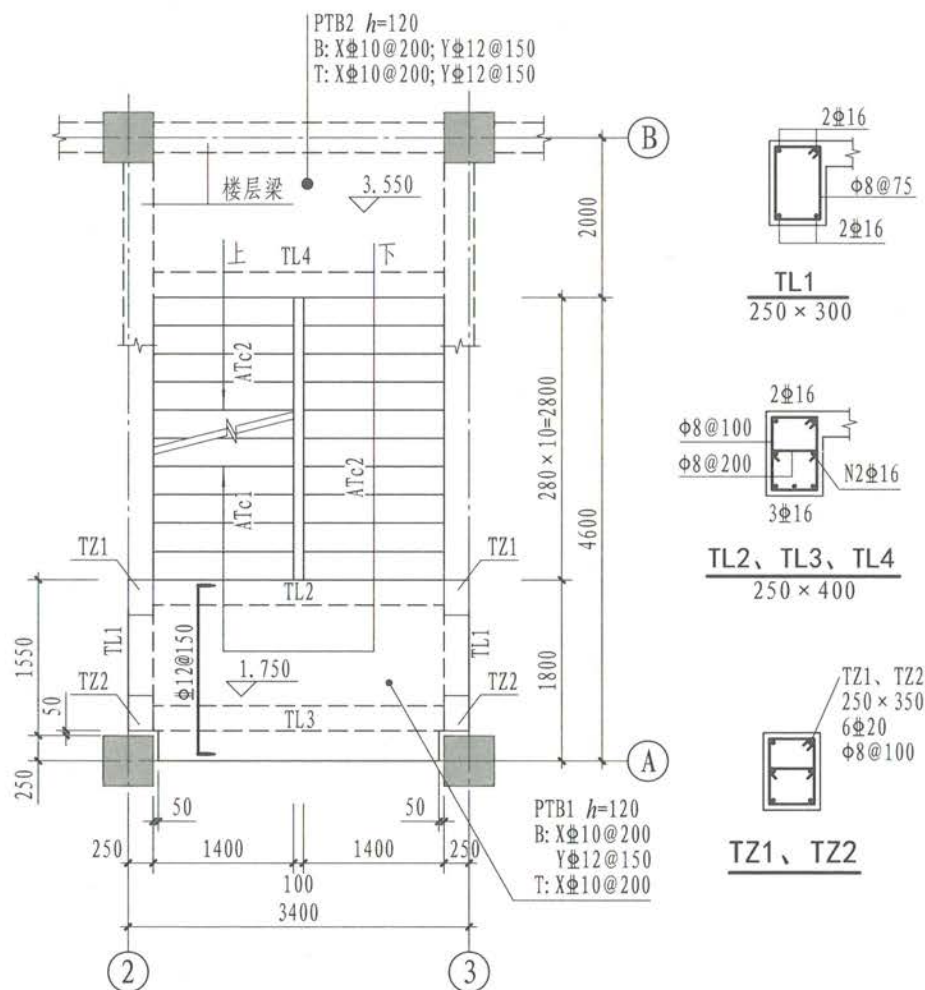
▽1.750~▽3.550楼梯平面图
