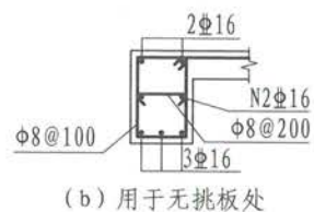
TL2、TL3、TL4 250 × 400
