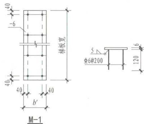
BTb、DTb型楼梯滑动支座构造详图
