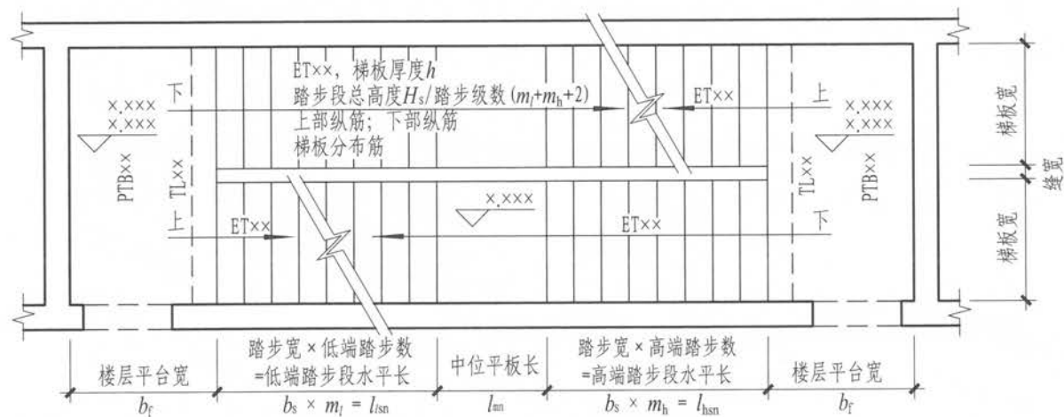
图1 \nabla x.xxx \sim \nabla x.xxx 楼梯平面图
