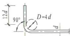
(a) 末端带90°弯钩
