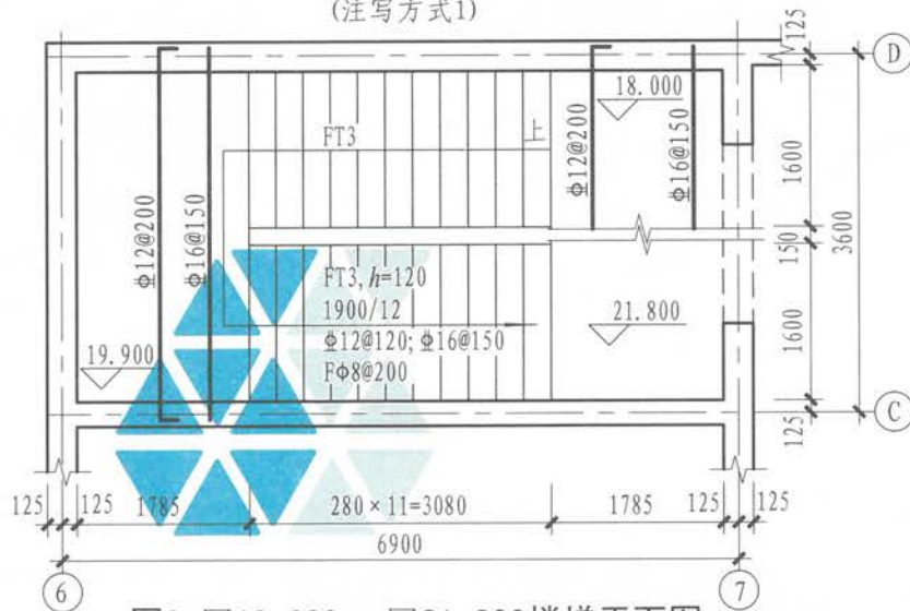
图3 ▽18.000~▽21.800楼梯平面图
