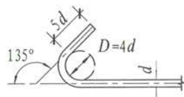
(b) 末端带135°弯钩
