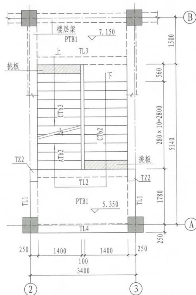
▽5.350~▽7.150楼梯平面图
